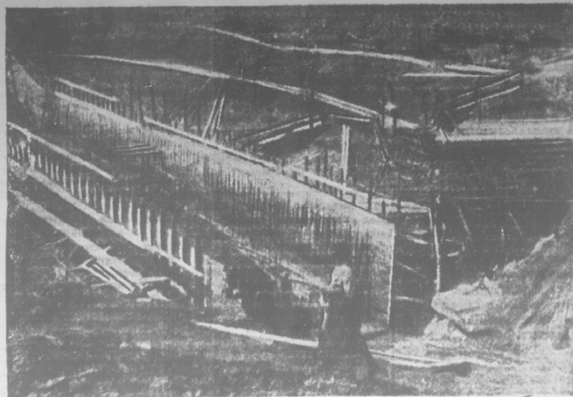
На 7-м километре трассы Невинномысского канала пересекает река Барсуцки. Здесь сооружается огромная железобетонная труба протяжением 150 метров. Дюкер пропустит воды канала и реки Барсуцки в свои прежние русла. На снимке: общий вид строительства. Фото Ю. Чечалина.
