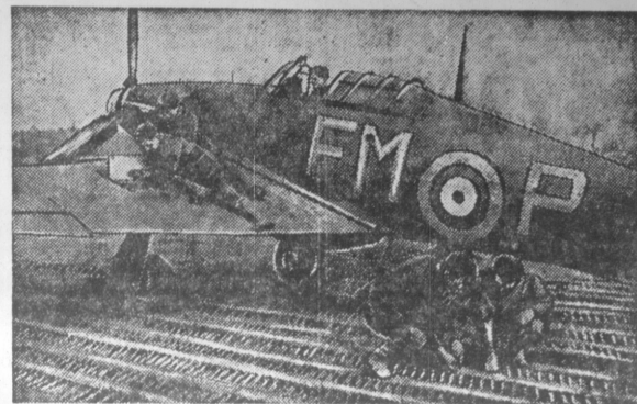
Военно-воздушные силы Англии. Разборная металлическая сетка, употребляемая на английских аэродромах для быстрого вылета самолета и приземления.
