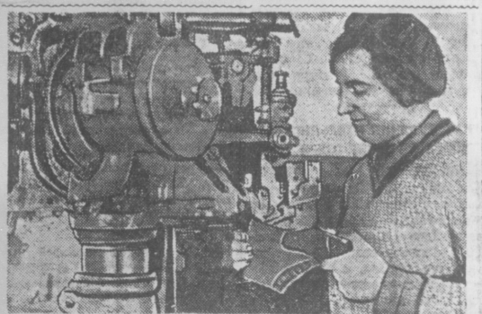
Работница Ворошиловской обувной фабрики Р. С. Ганза, сменяющая товарища, ушедшего в Красную Армию, успешно овладела процессом работы на сложной машине. На снимке: тов. Ганза за работой.
