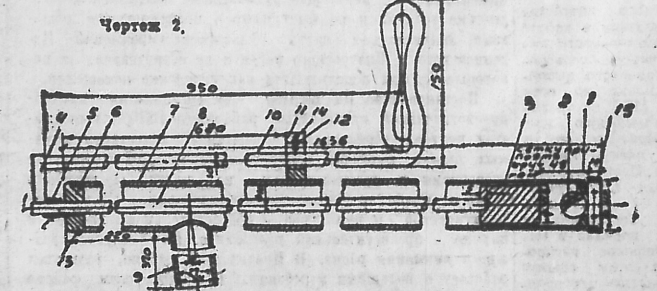
ТРУБНЫЙ НАСОС: 1 — Гнездо клапана, 2 — шарик, 3 — поршень, 4 — стойка приводной штанги, 5 — пружина, 6 — крышка, 7 — цилиндр, 8 — шток, 9 — выводящий патрубок, 10 — приводная тяга, 11 — наравляющая вилка, 12 — шпилька, 13 — шуруп, 14 — шпатель, 15 — фильтрующая сетка. (9), представляющий собой кусок трубы с внутренним диаметром 26 — 27 мм. Поршень — (3) изготавливается из круглого железа, диаметр его — 34,5 мм. К поршню приварен шток — (8), который верхним концом проходит через крышку насоса. К верхнему концу штока приваривается стойка приводной тяги — (4), к которой в свою очередь приварена приводная тяга — (10). Для направления движения приводной тяги к цилиндру приварена направляющая вилка — (11). Чтобы избежать ударов стойки о крышку, между ними ставят
