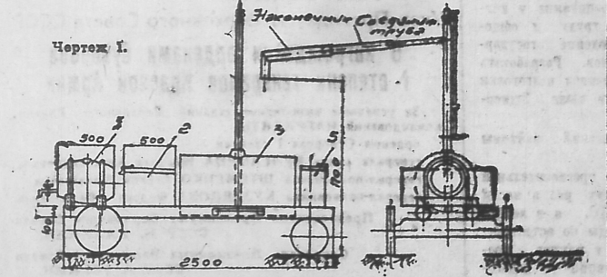
ЗАПРАВочная тележка с трубным насосом. СМОНТИРОВАНЫ НА КРЕСТЬЯНСКОМ ХОДУ: 1 — Бочка для отработавшего автоса, 2 — ящик для заправочного инвентаря, 3 — бочка для горючего, 4 — насос, 5 — дополнительный ящик.
