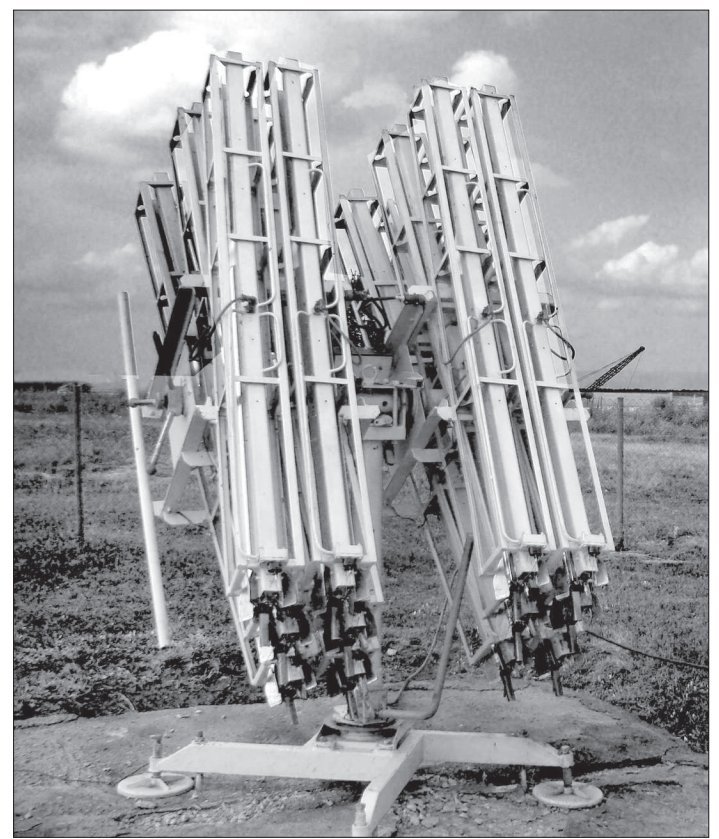
При помощи таких установок на Ставрополье расстреливают градовые облака.
